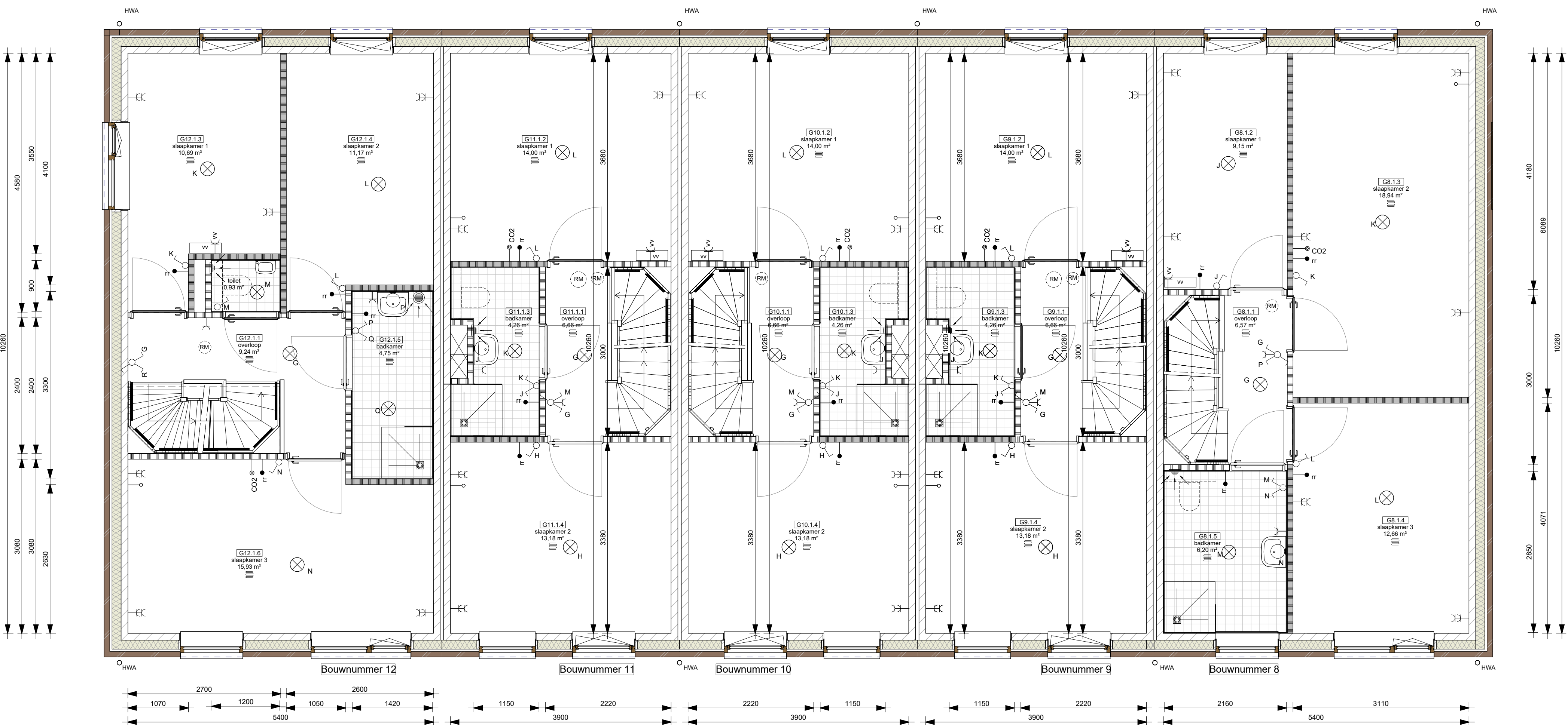
Tweede verdieping
