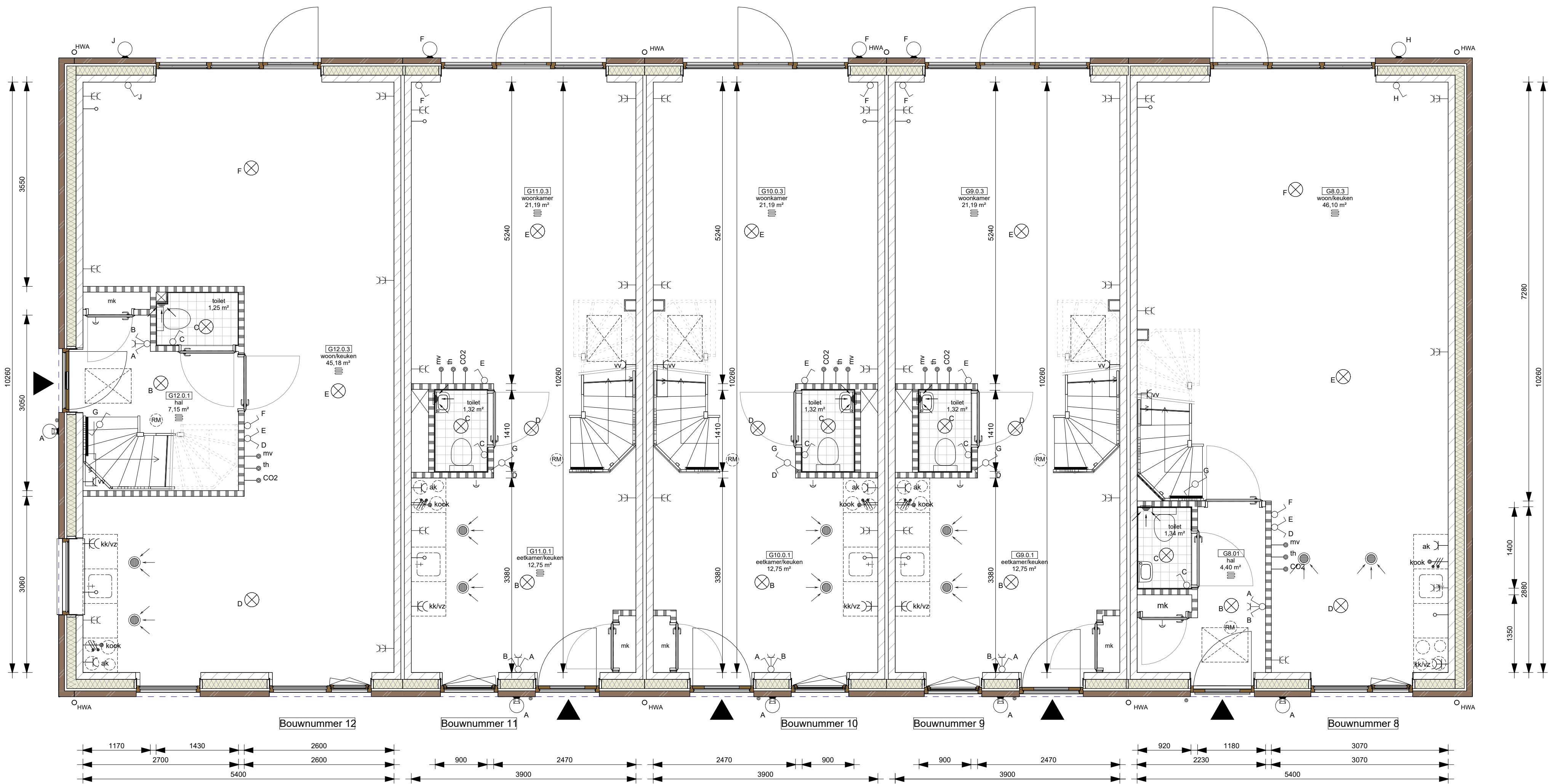
Begane grond
