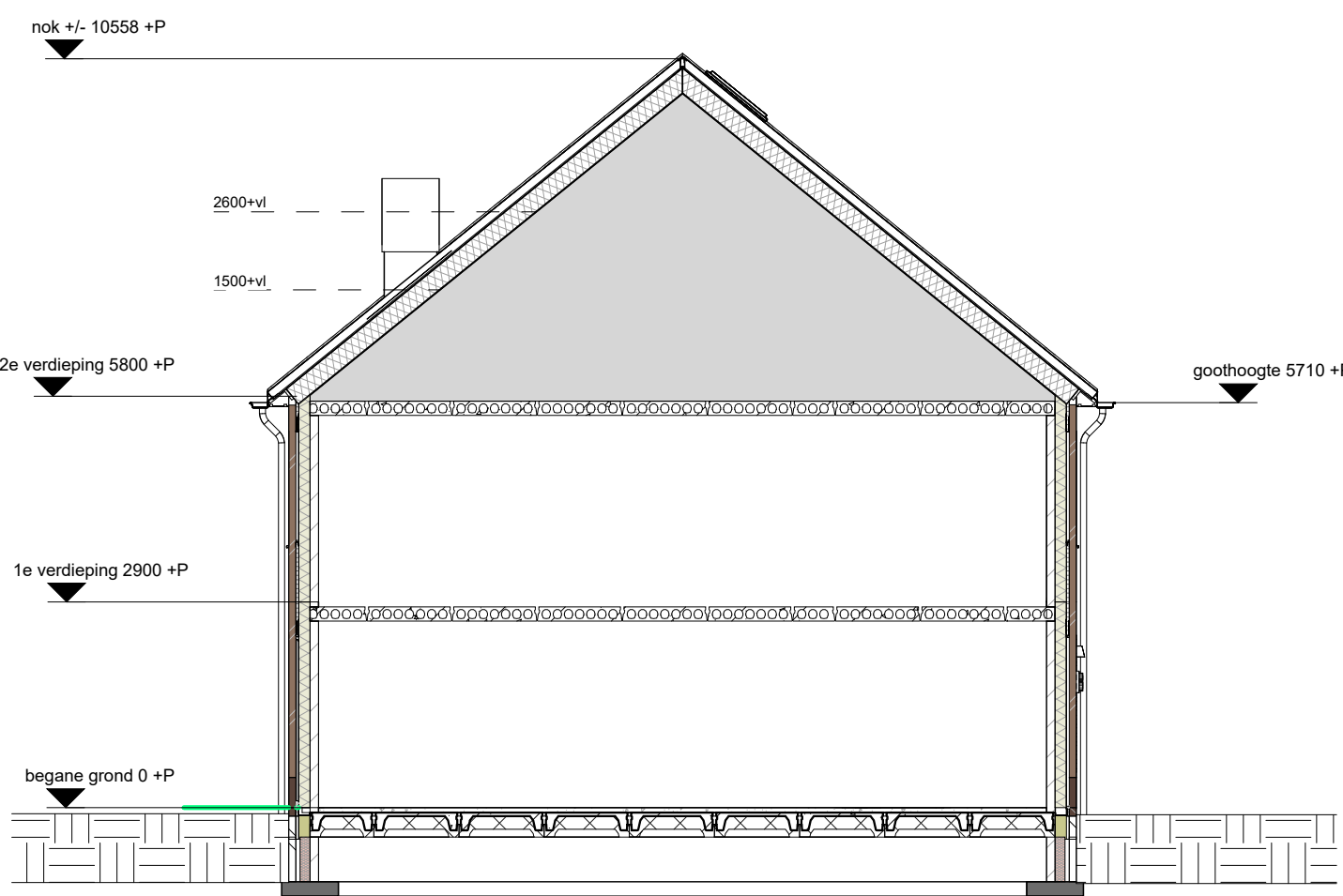
Dwarsdoorsnede
